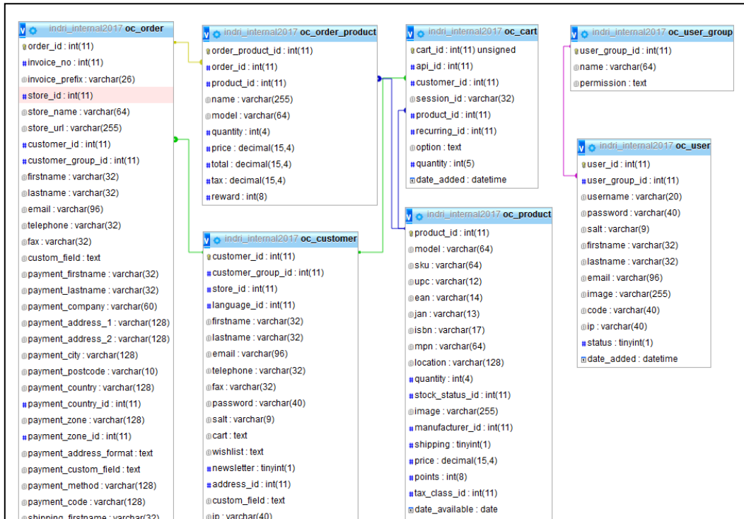
Gambar 2 Desain Konseptual Database
