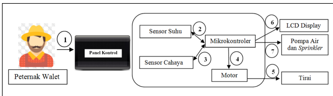
Gambar 2. Sistem Pengontrolan Suhu dan Intensitas Cahaya
