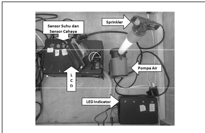
Gambar 6. Implementasi Perangkat Keras Sistem Pengontrolan Suhu dan Intensitas Cahaya
